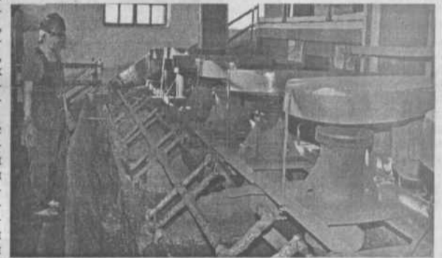
Отделение флотации фабрики.
