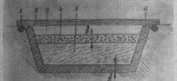
Схема закладки парника отбросов и нечистот для обезвреживания: 1. Отбросные рамы парника. 2. Рама парника, покрытая стеклом или полиэтиленовой пленкой. 3. Воздушное пространство. 4. Слой почвы. 5. НАВОЗ, нечистоты, мусор, заложённые для обезвреживания и как биотермическое топливо. 6. Слой жирной, мятой и утрамбованной глины.
