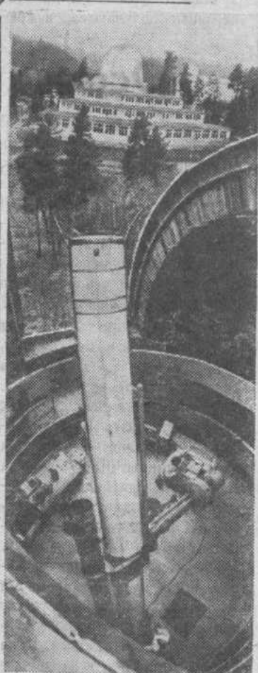
Грузинская ССР. На снимке: сорокасантиметровый телескоп-рефрактор Абастуманской астрофизической обсерватории.
