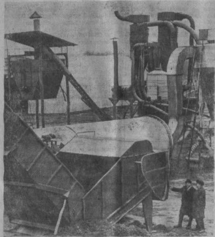
НА СНИМКЕ: технологическая линия для приготовления и брикетирования кормов.
