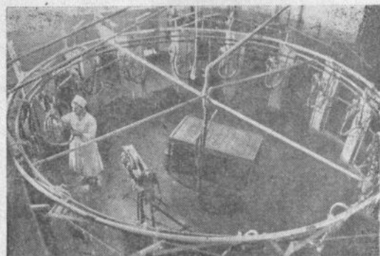
ОРЕНБУРГСКАЯ ОБЛАСТЬ. В колхозе имени Максима Горького Новосергиевского производственного управления работает доильная установка типа «карусель», способная пропустить за смену 500 коров. Доильный зал оборудован молокопроводами, сепараторами, системой очистки и охлаждения молока.
