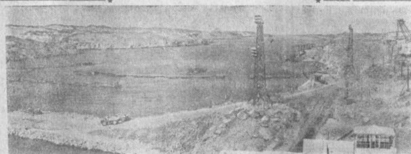
На строительстве высотной Асуанской плотины в Объединенной Арабской Республике. Перекрытие Нила состоится 15 мая. В этот день каменно-песчаная плотина навсегда перегородит старое ложе реки. Могучий Нил понесет свои воды по новому руслу — обводному каналу.
